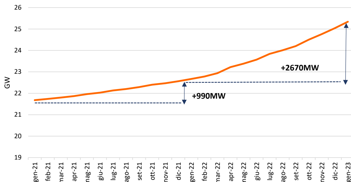
Fig.1.8: Trend di installazione di nuova capacità fotovoltaica
