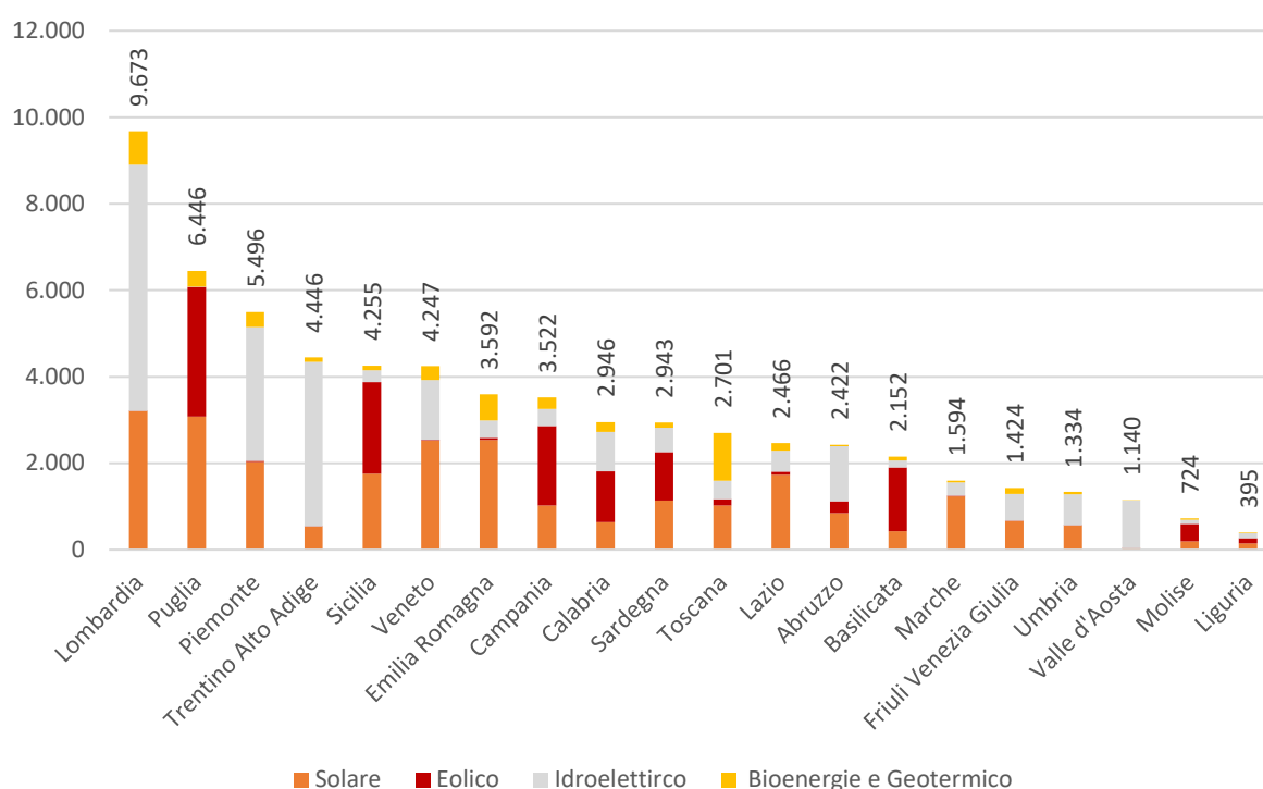
Fig.1.7: Capacità di generazione elettrica per tecnologia (MW, dati al 31/01/2023)
